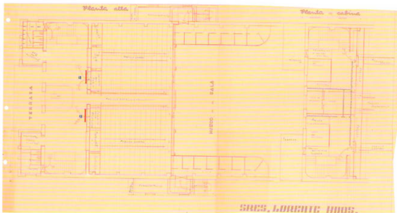
Teatro Requena. Planta alta y cabina
