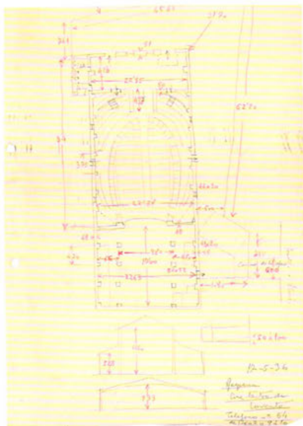
Teatro Circo Requena. Croquis con cotas planta, alzado y sección
