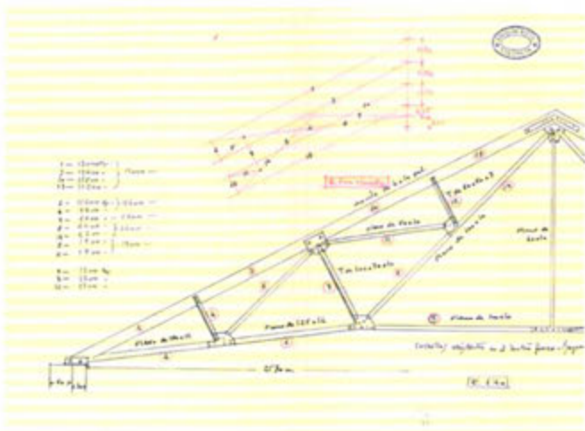
Cuchillo. Teatro Circo Requena. Plano de cubierta, escala 1:40
