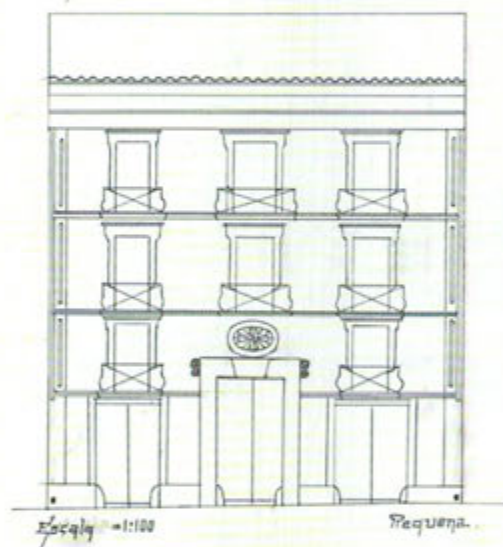
Navarro Generalísimo 37 alzado y plano distribución Escala 1.100
