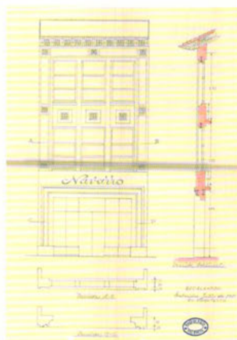
Edificio Navarro Alzado y secciones AB CD 1.50
